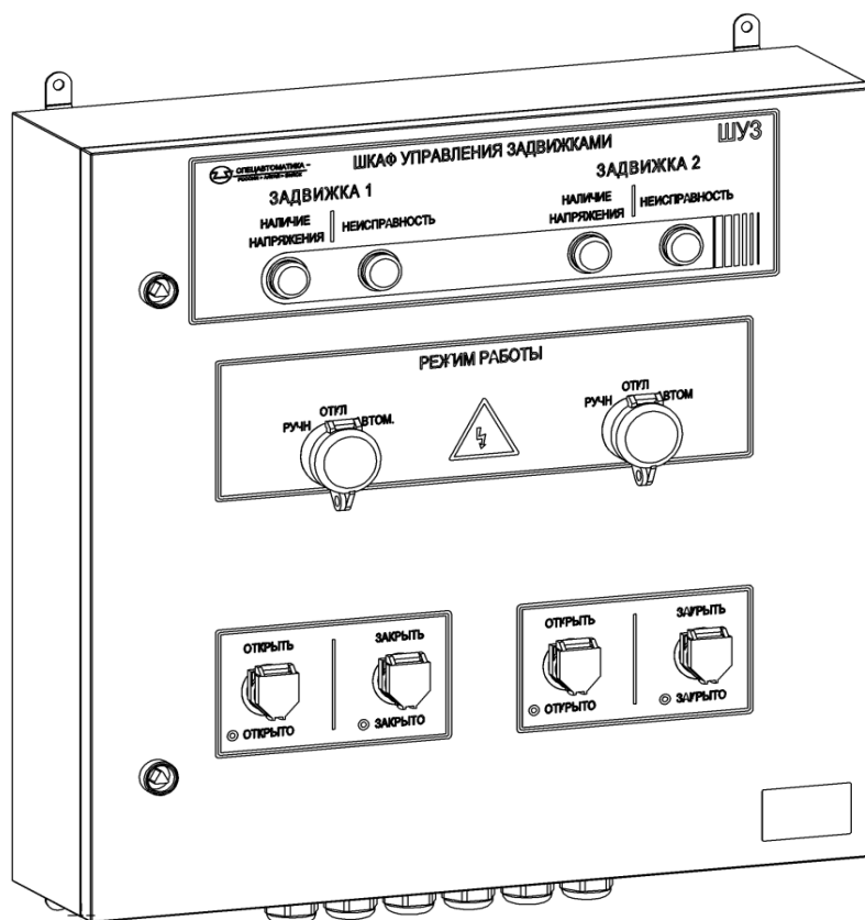
Рисунок 1-Общий вид шкафа
