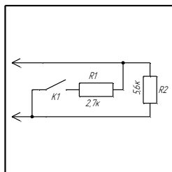
Переключательный контакт с контролем целостности цепи (тип 2)
