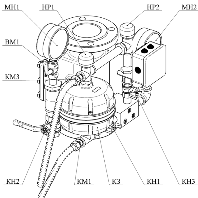
Узел управления sprinkлерный водозаполненный с камерой задержки
