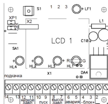
Расположение клемм и микроджамперов
