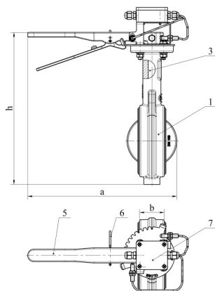
«АМК», DN 125(150) с УКП3А V1; V2
