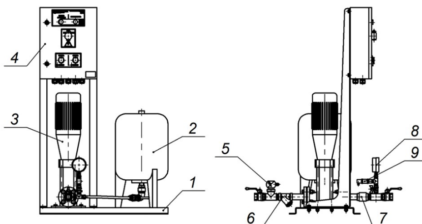
Рисунок 1 — Общий вид жокей-насоса с мембранным баком
