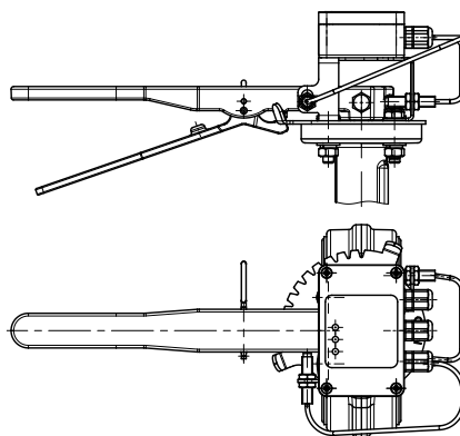
«АМК», DN 125(150) с УКП3А V3
