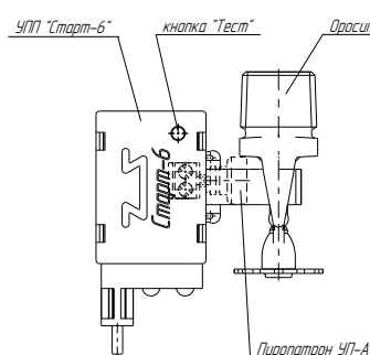
Схема установки УПП «Старт-6» на ороситель
