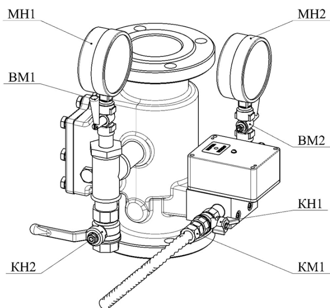
Узел управления sprinkлерный водозаполненный с устройством задержки
