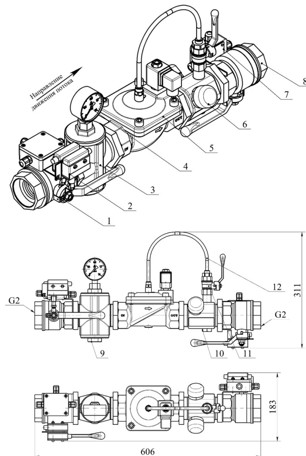
Рисунок 1 - Общий вид, габаритные и присоединительные размеры УУ дренчерного с электроприводом «Малорасходный»
