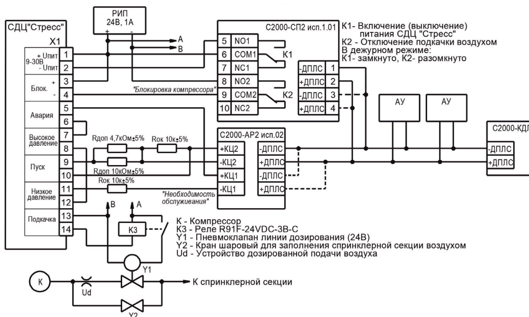
Схема СДЦ «Стесс» к С200-КДЛ (С2000-СП2 вер.1.01, С2000-АР2 исп.02
