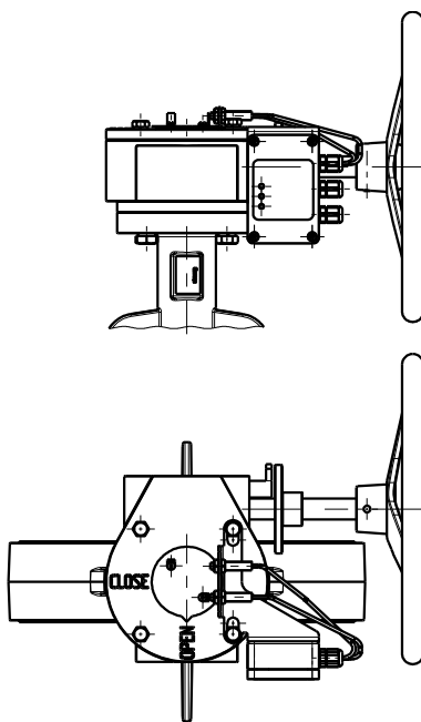
«АМК», DN 200(250) с УКП3А v3
