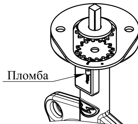
Опломбированный затвор
