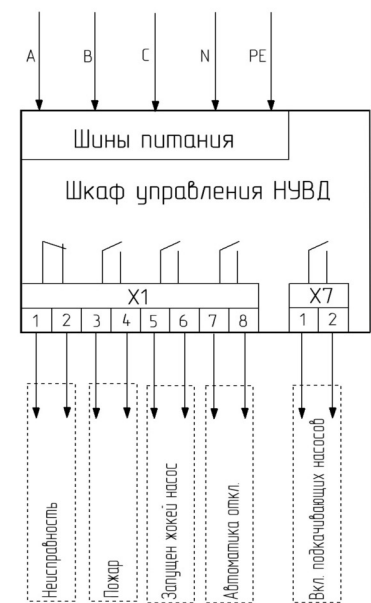
Схема внешних подключений
