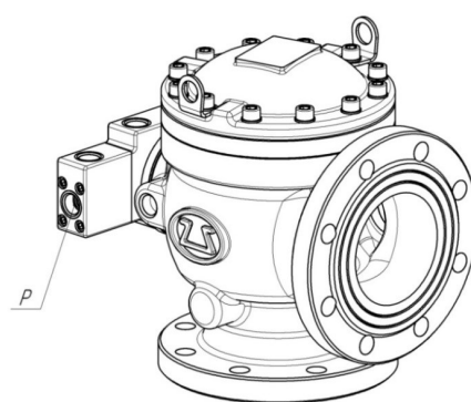
Рисунок 2 - Общий вид клапана КСД типа КМУ
