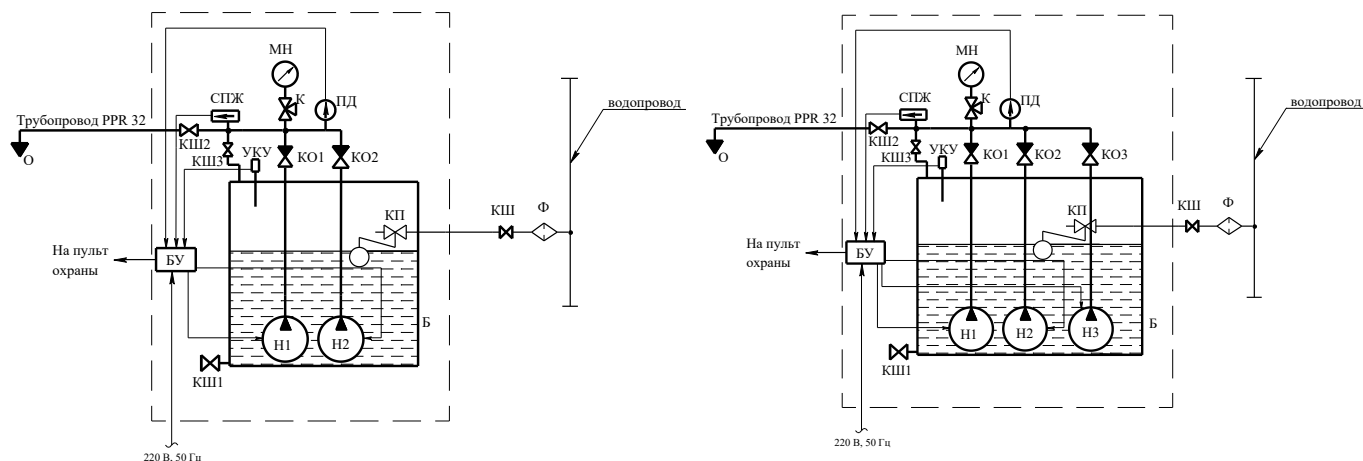
Рисунок 2—Схема функциональная системы спринклерного пожаротушения на основе МПОВ 500.2 (пример)
