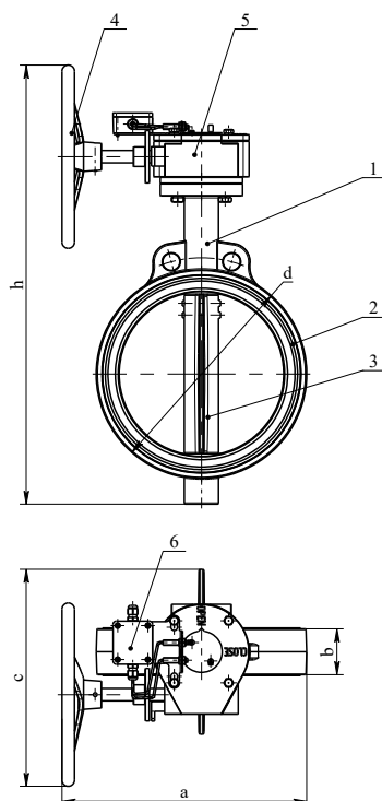
«АМК», DN 200(250) с УКП3А v1, V2
