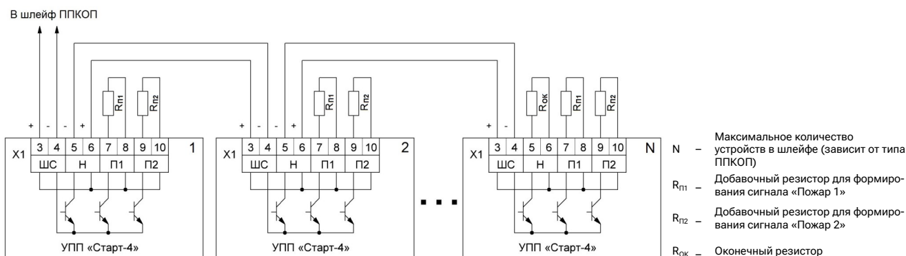
Схема подключения устройств в шлейф пожарной сигнализации
