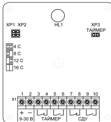
Рисунок 1-Печатная плата модуля УУ с устройством задержки с расположением клемм и перемычек (диаметр кабеля для подключения должен быть в пределах от 4 до 7 мм, сечение подключаемых проводников кабеля должно быть не более 2,5 мм)
