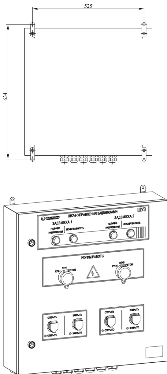
Рисунок 1 — Общий вид шкафа
