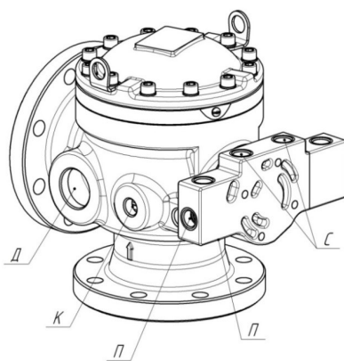
Рисунок 2 - Общий вид клапана КСД типа КМУ
