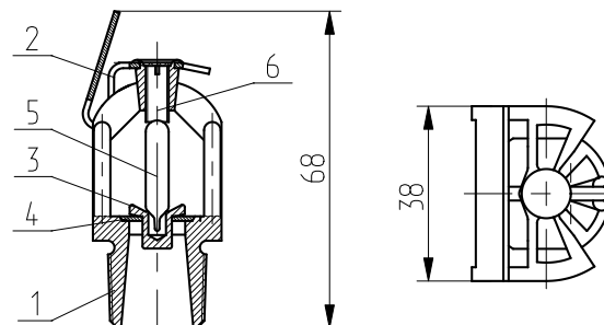
Рисунок 1 – Состав оросителя
