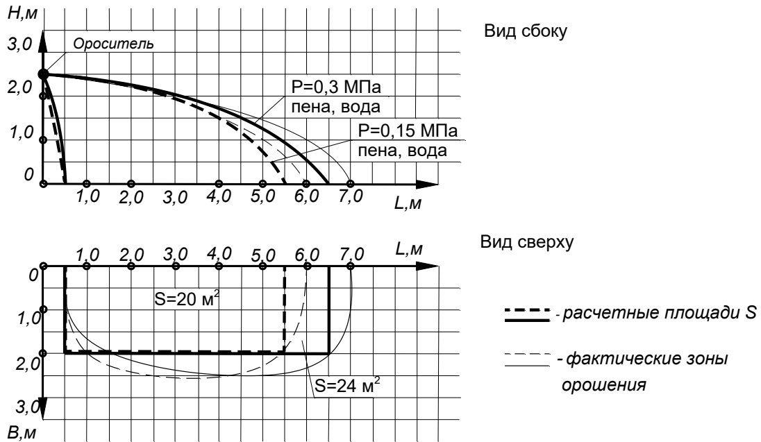
Карта орошения ОТВ оросителей «СВГ-15», «ДВГ-15» при установке вертикально розеткой вниз для создания водяной завесы
