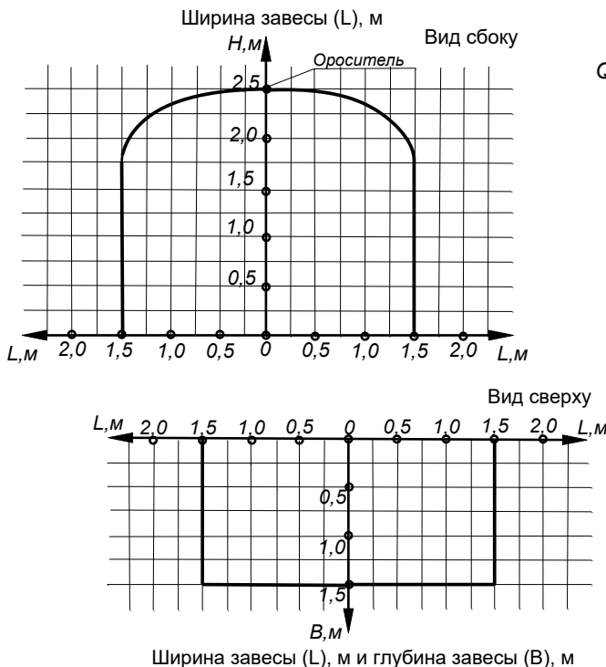
Карта орошения ОТВ оросителей «СВГ-15», «ДВГ-15» при установке вертикально розеткой вниз для создания водяной завесы
