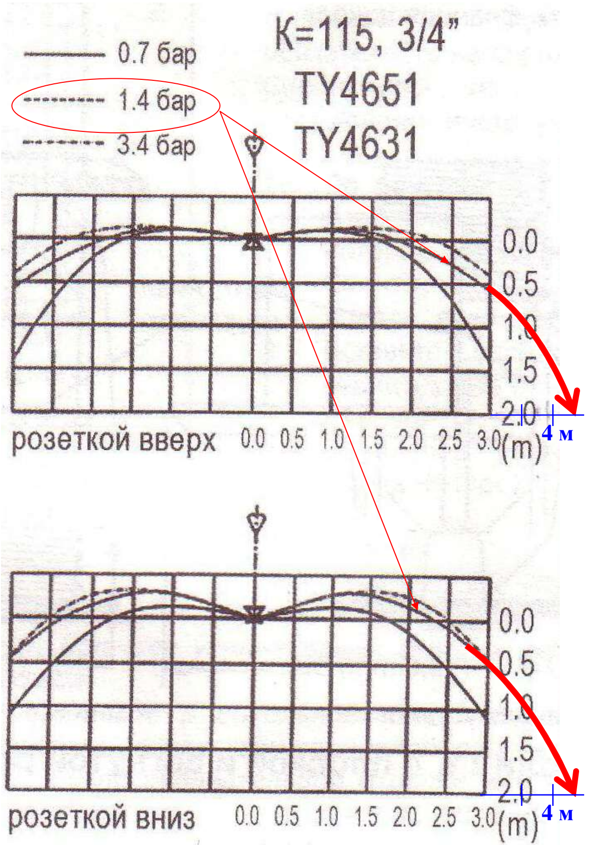
Рис. 2 Эпюра «ТУ 4651»
