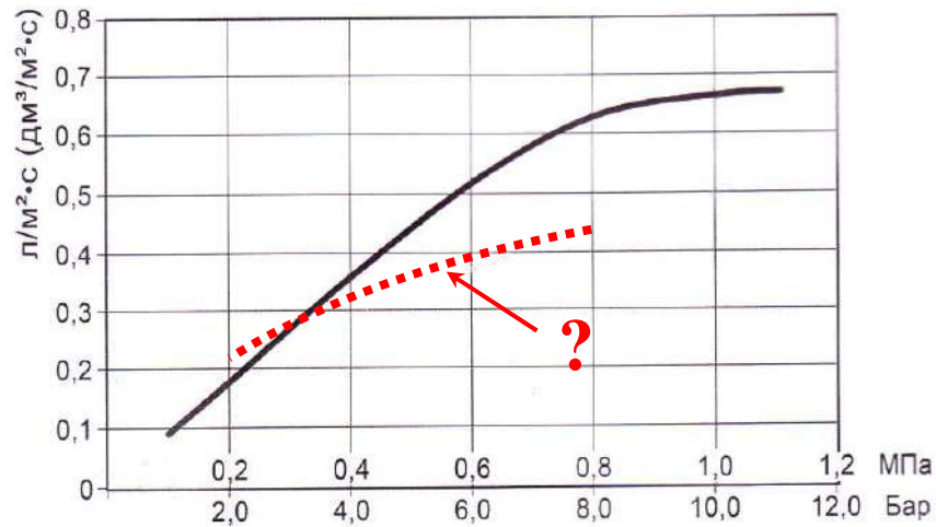
Рис. Е Для оросителей ТУ4251/ТУ4231 График зависимости интенсивности орошения от давления (ГОСТ Р 51043-2002)
