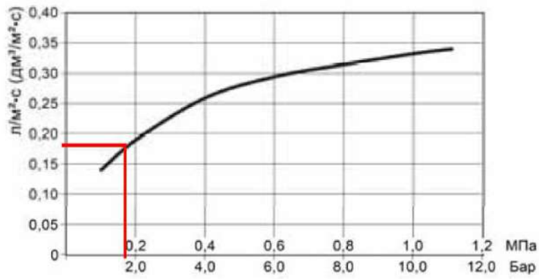
Рис. 3 График «ТУ 4651»
