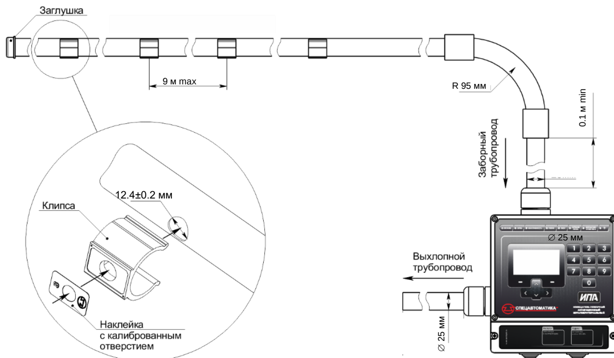
Рисунок 12 – Подключение воздухозаборной системы
