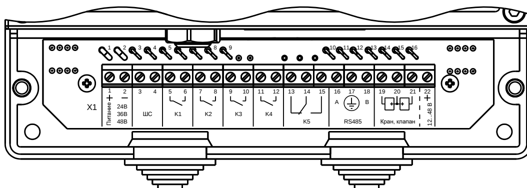
Рисунок 15 – Клеммы извещателя
