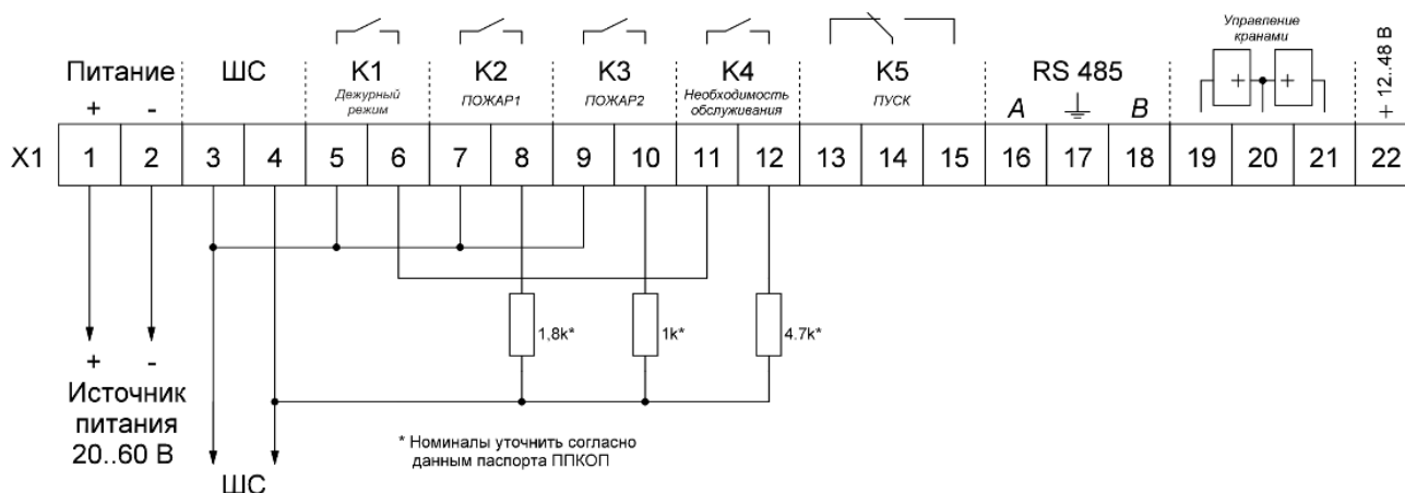
Рисунок 17 – Схема подключения с обобщенным сигналом об обслуживании
