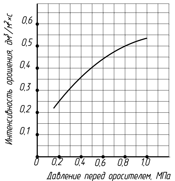
Ороситель "ОЭ-25"
