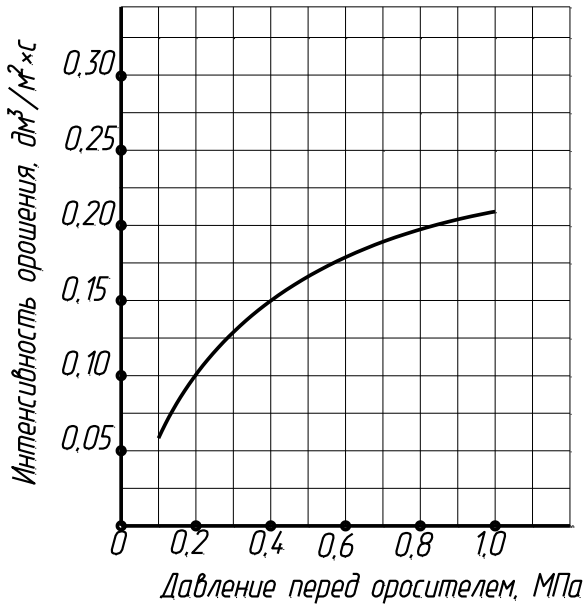
Ороситель "ОЭ-16"
