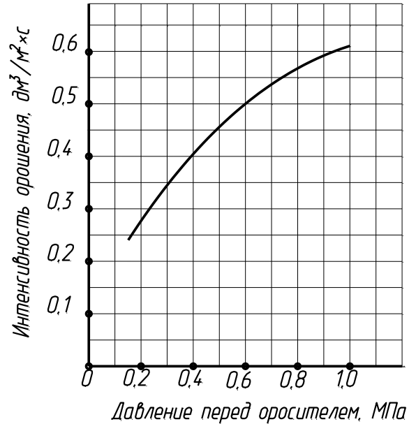
Ороситель "ОЭ-25"
