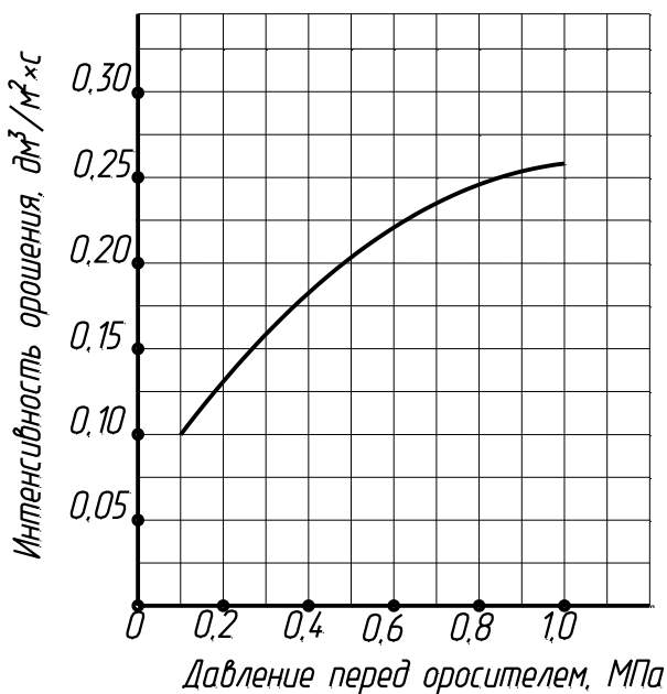
Ороситель "ОЭ-15"
